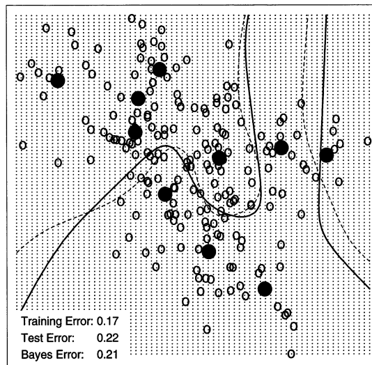
MDA - 5 Subclasses per Class
